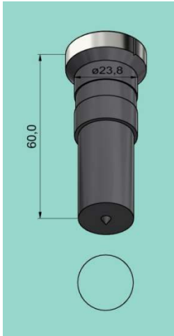
Rundstempel APS 23
