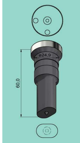
Langlochstempel APS 24
