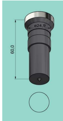
Rundstempel APS 24
