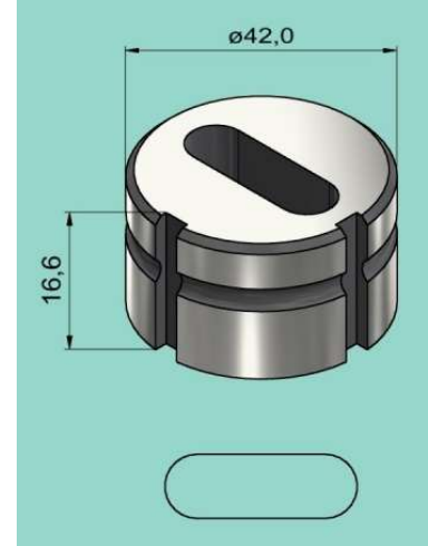
Langlochmatrize APS 42
