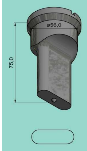
Langlochstempel PL
