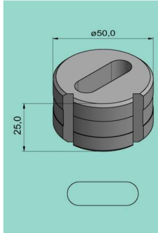
Langlochmatrize MS
