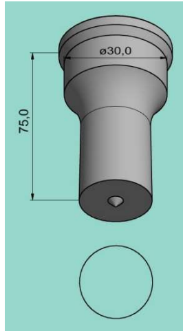
Rundstempel PM
