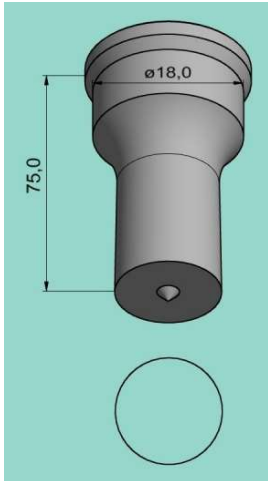
Rundstempel PS
