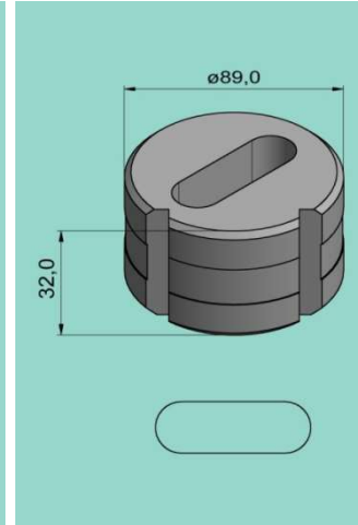
Langlochmatrize MM
