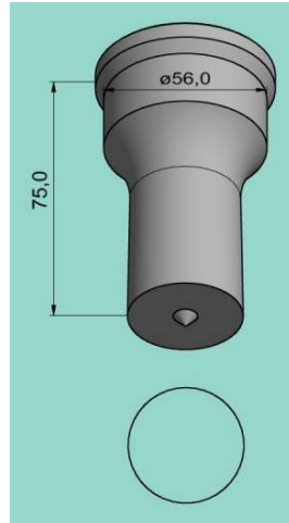
Rundstempel PL
