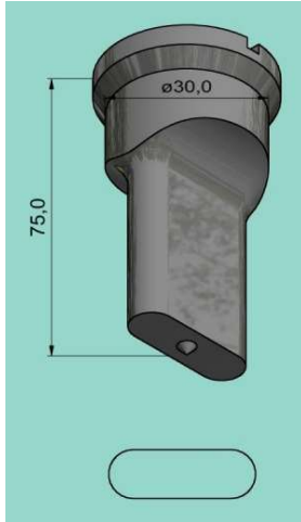
Langlochstempel PM
